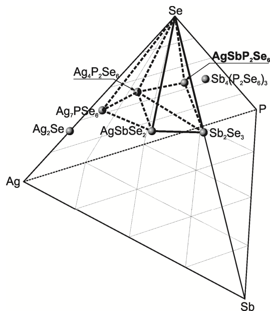
Рис. 1. Квазібінарні системи \text{Ag-Sb-P-Se} встановлені за даними [11].
